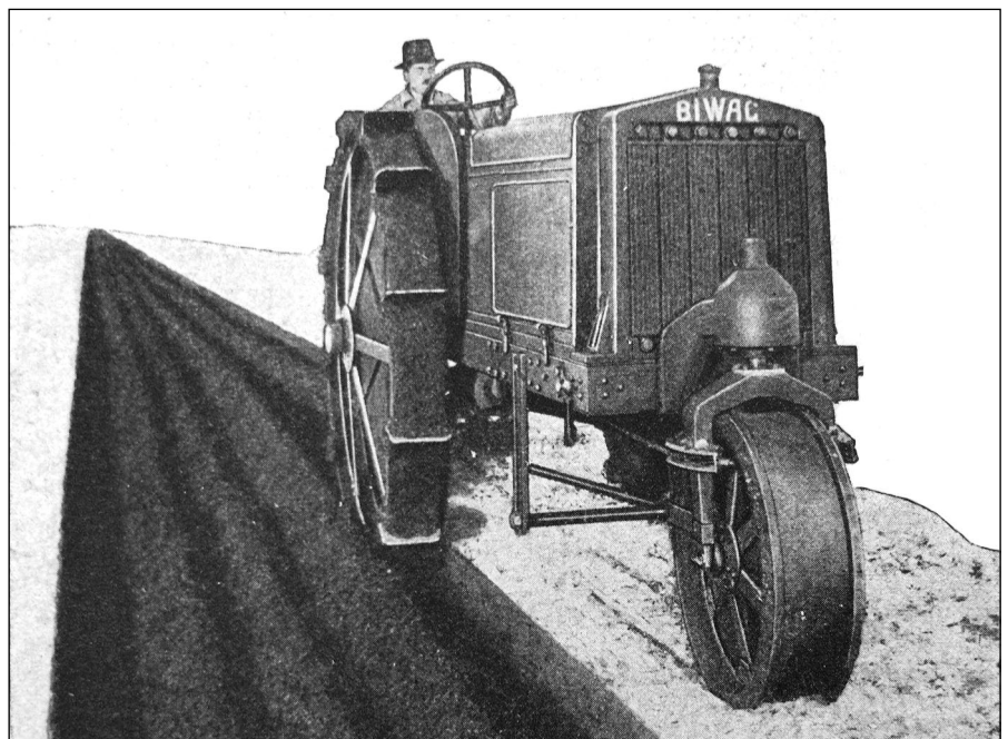
Biwag-Motorpflug (System Eickemeyer)1920 1
