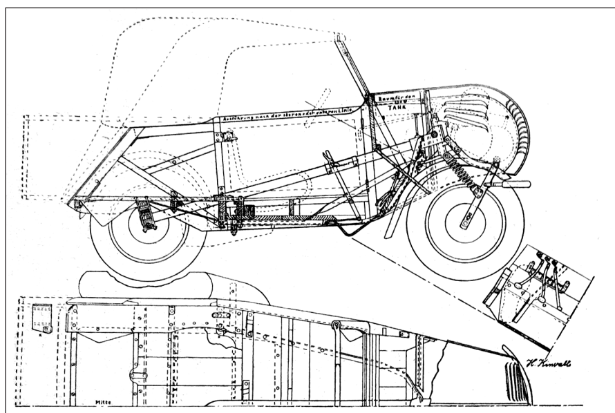
Das Hjaki-Dreirad nach einer Zeichnung des Entwicklers H. Kinvall 1
