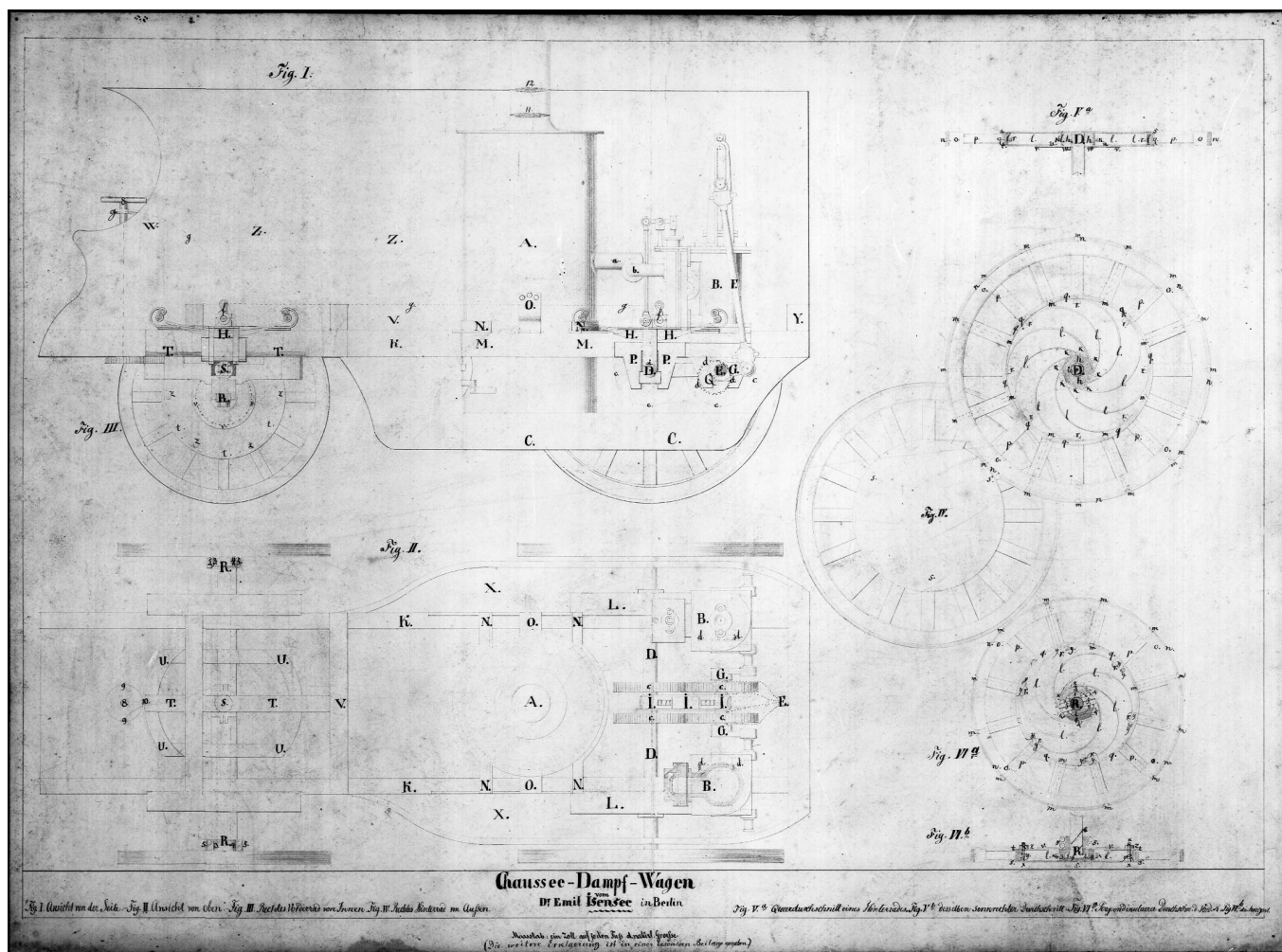
Funktions-Zeichnung des Dampf-Chaussee-Wagens von Dr. Emil Isensee von 1838
