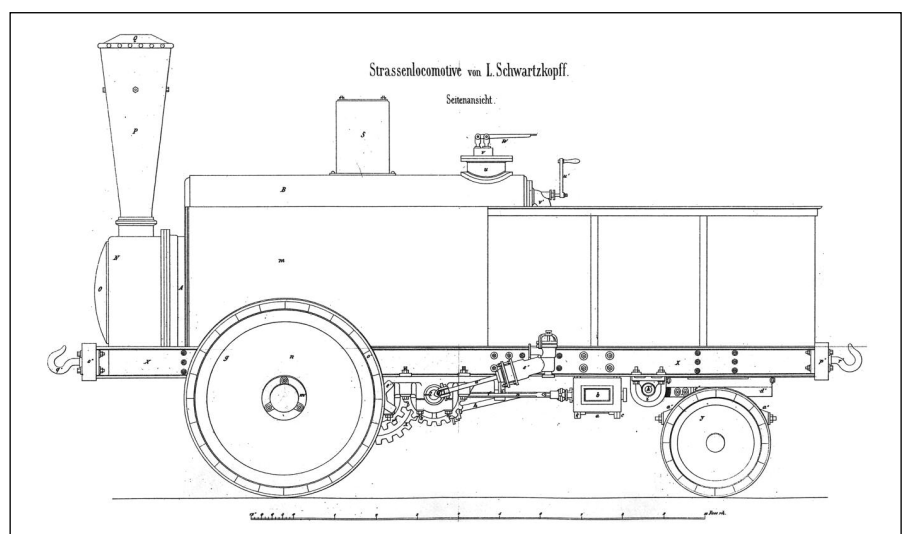
Konstruktion des Dampfwagens System Schwartzkopff von 1863
