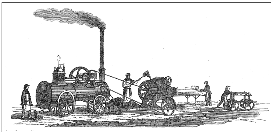
Eine Wens-Lokomobile treibt 1862 eine Ziegelpressmaschine der Gebr. Sachsenberg an 1
